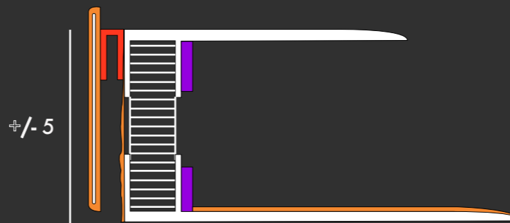
aggancio in estensione (sezione)
