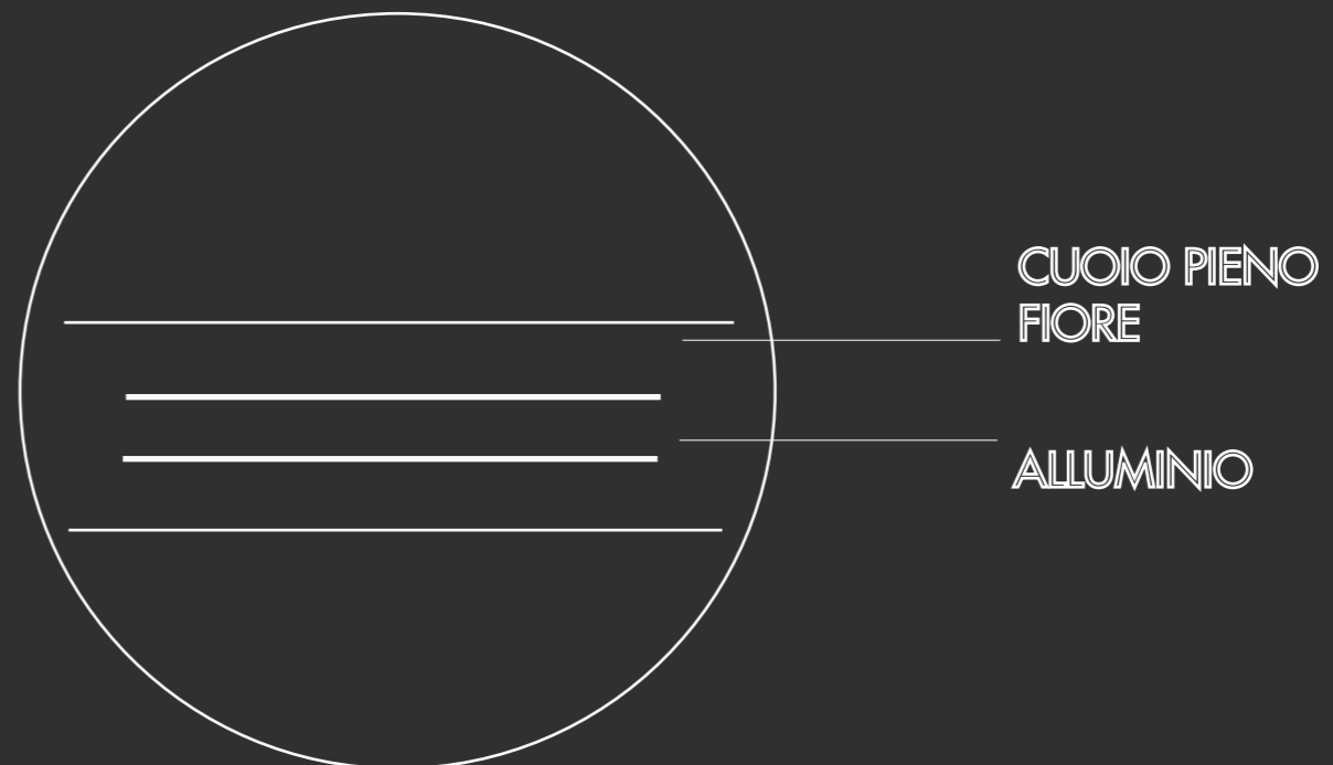
SEZIONE
